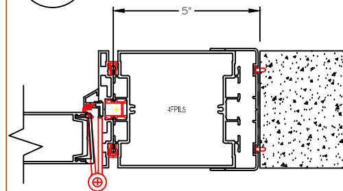
DF @ 5" Mini-End Aluminum Door
